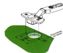
Установка дверей
