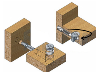
Евровинт 7 x 50
